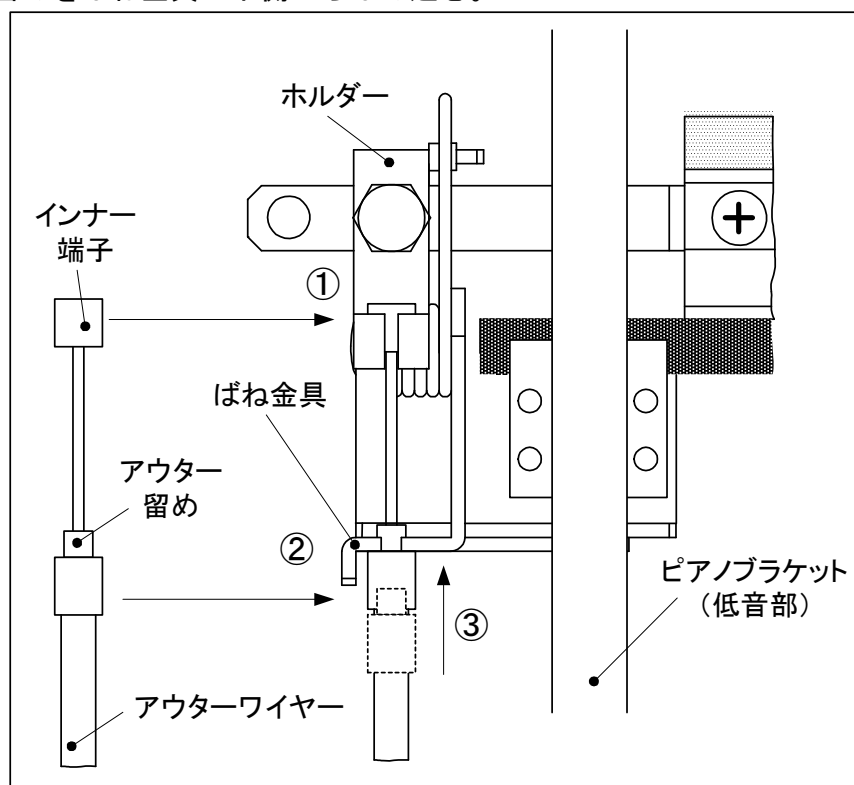
図3.3-3 ワイヤーの掛け方
